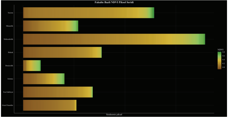
Şekil 8. Fakülte düzeyinde NDVI piksel şeridi
