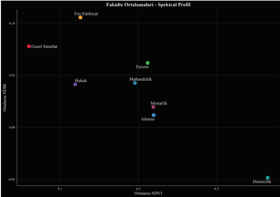
Şekil 6. Fakülte düzeyinde spektral ortalamalar (yatay eksen ortalama NDVI, dikey eksen ortalama NDBI)
