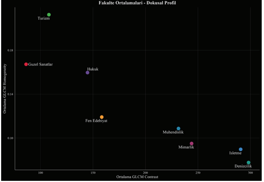
Şekil 7. Fakülte düzeyinde dokusal ortalamalar (yatay eksen ortalama GLCM kontrast, dikey eksen ortalama GLCM homojenlik)
