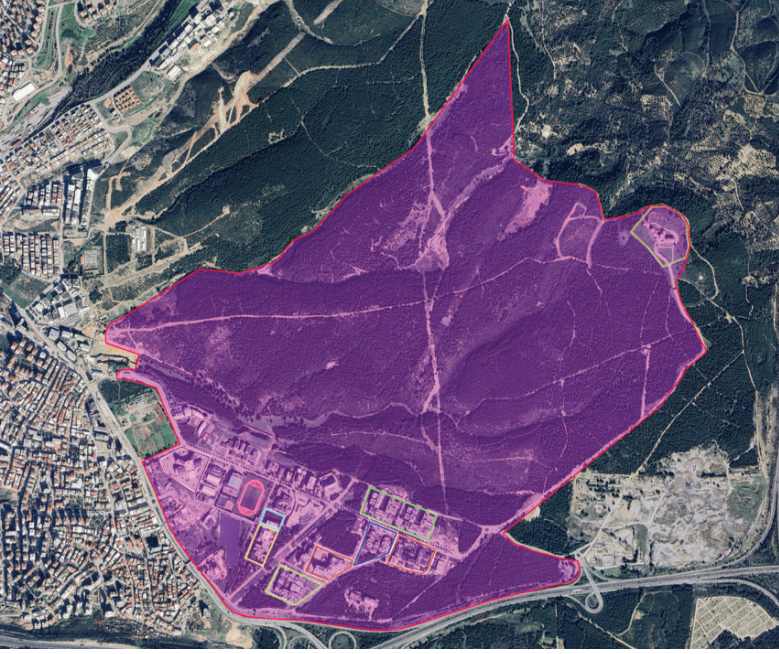
Şekil 2. DEÜ Merkez Kampüsü sınırı ve sekiz fakülte poligonunun Sentinel-2 görüntüsü üzerindeki konumları (Copernicus Sentinel-2, 2021). Görüntü tarihi: 24/08/2024.
