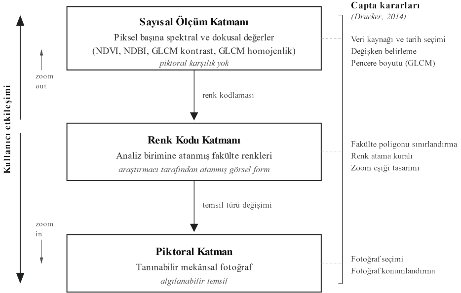
Şekil 3. Katmanlı temsil modelinin kavramsal yapısı
