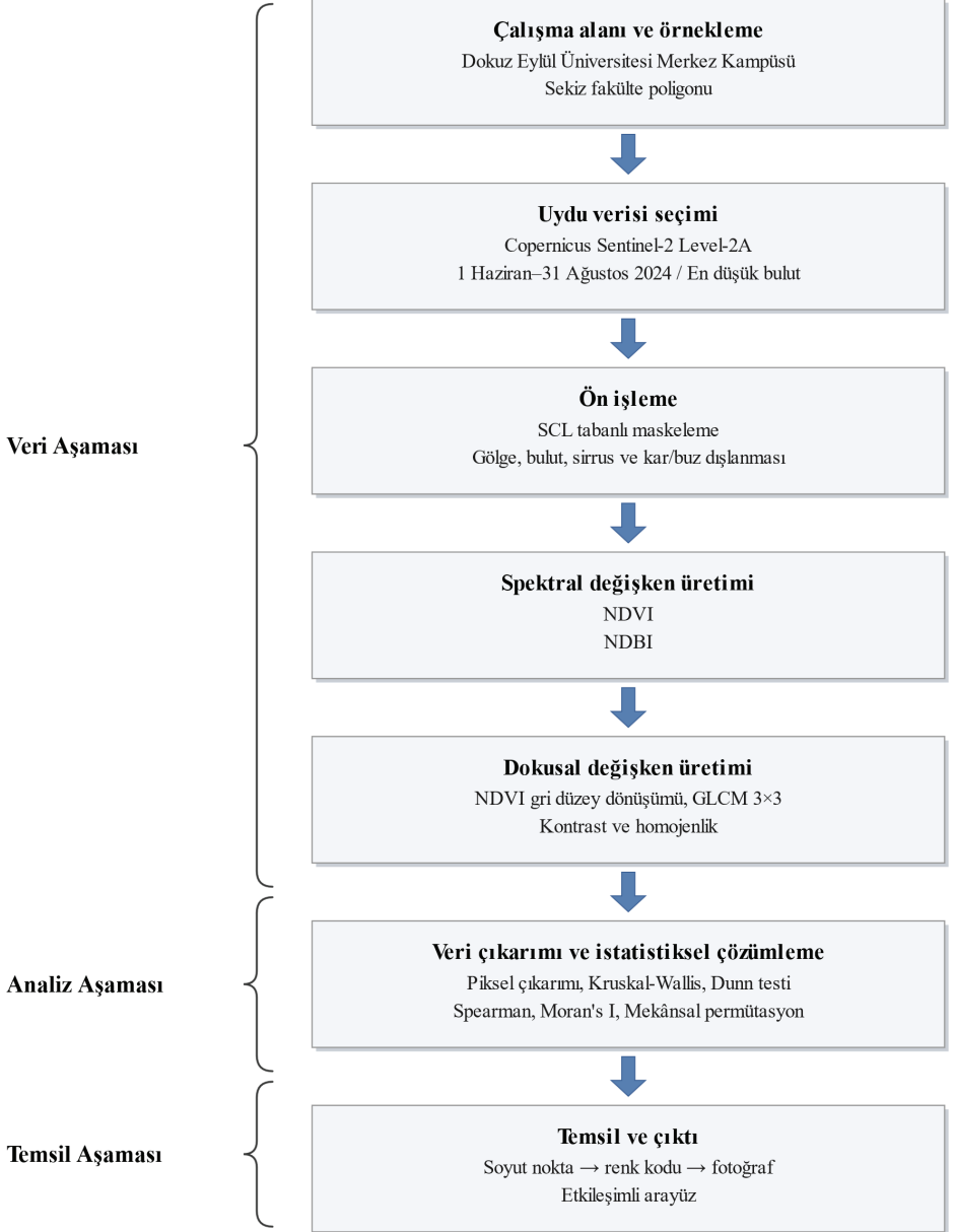
Şekil 1. Çalışmanın yöntemsel akışı ve süreç aşamaları
